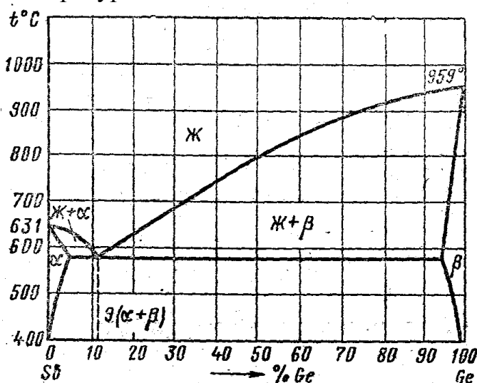
Рисунок – Диаграмма состояния Sb – Ge
