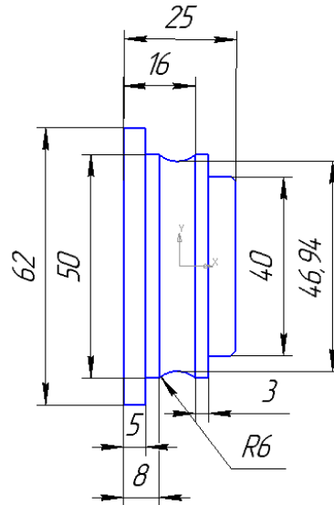
Рисунок 1 — Эскиз детали, обрабатываемой фасонным резцом
