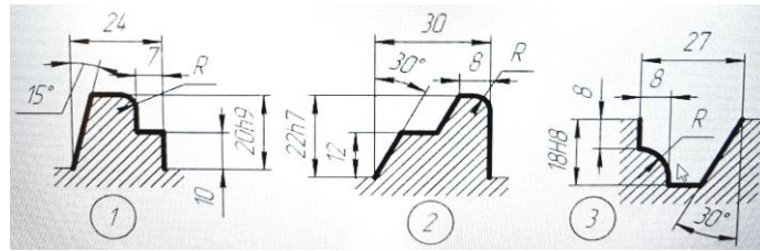
Рисунок 2 — Эскизы деталей для проектирования набора фрез.
