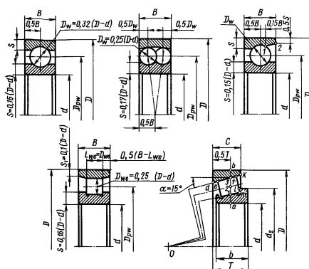
Рисунок 1 — Размеры подшипников к практическому занятию 1
