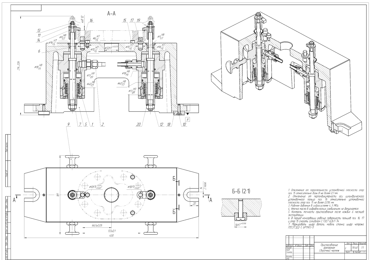
Рисунок 8 — Сборочный чертёж станочного приспособления
